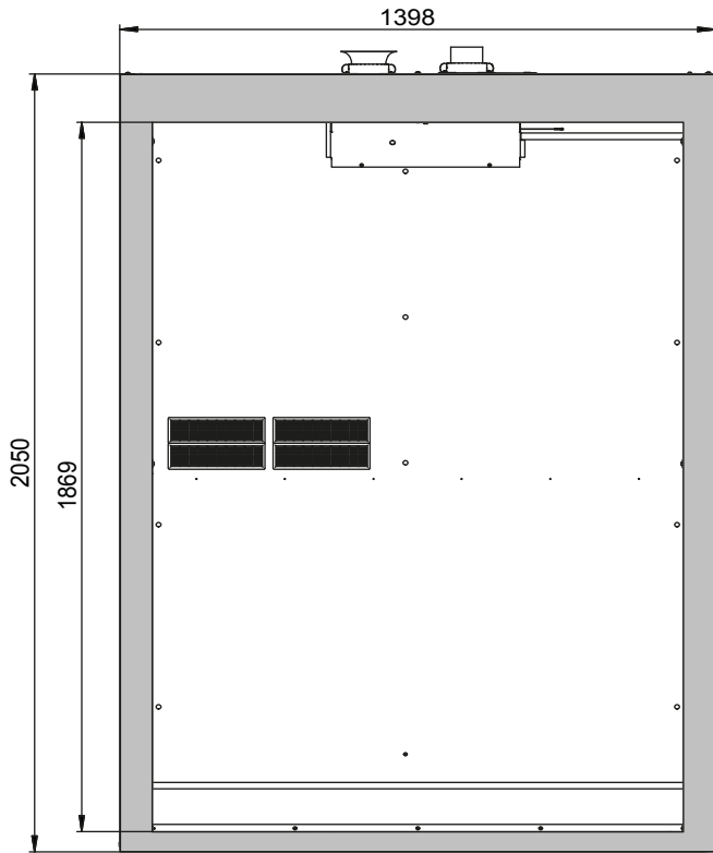
Vooranzicht
