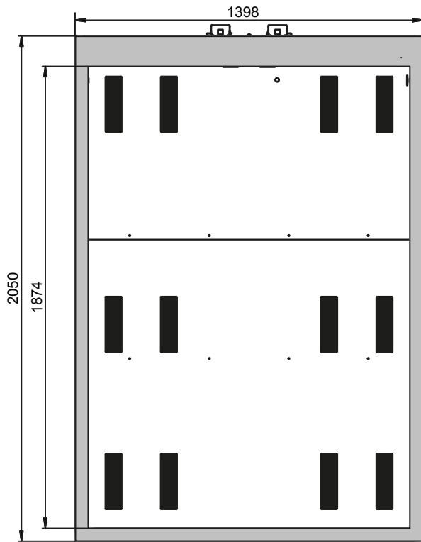
Vooraanzicht
