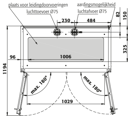
Bovenaanzicht
