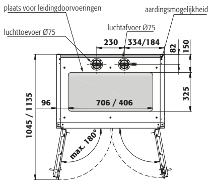
Bovenaanzicht
