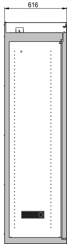
Zijaanzicht
