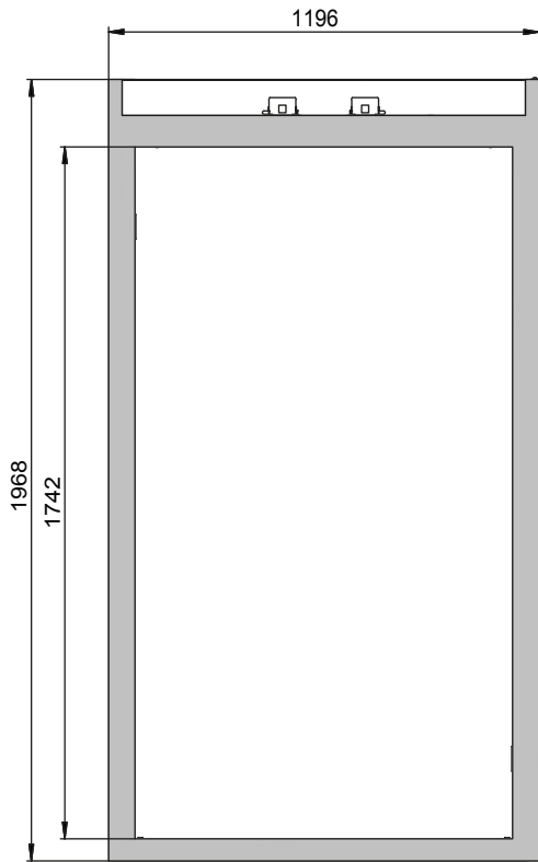
Vooraanzicht
