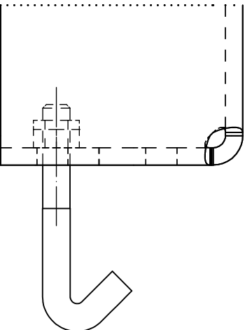
Detail2 Maßstab 1:1,5
