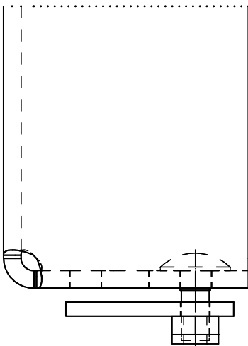
Detail1 Maßstab 1:1,5
