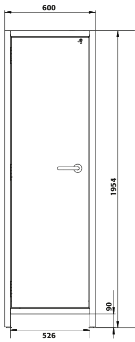
Vooranzicht
