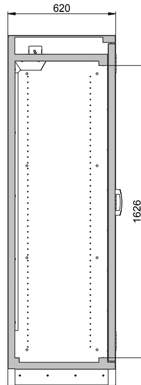
Zijaanzicht
