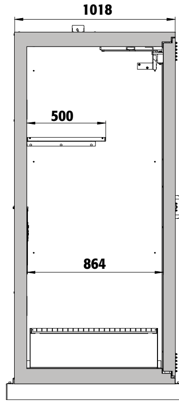
Zijaanzicht
