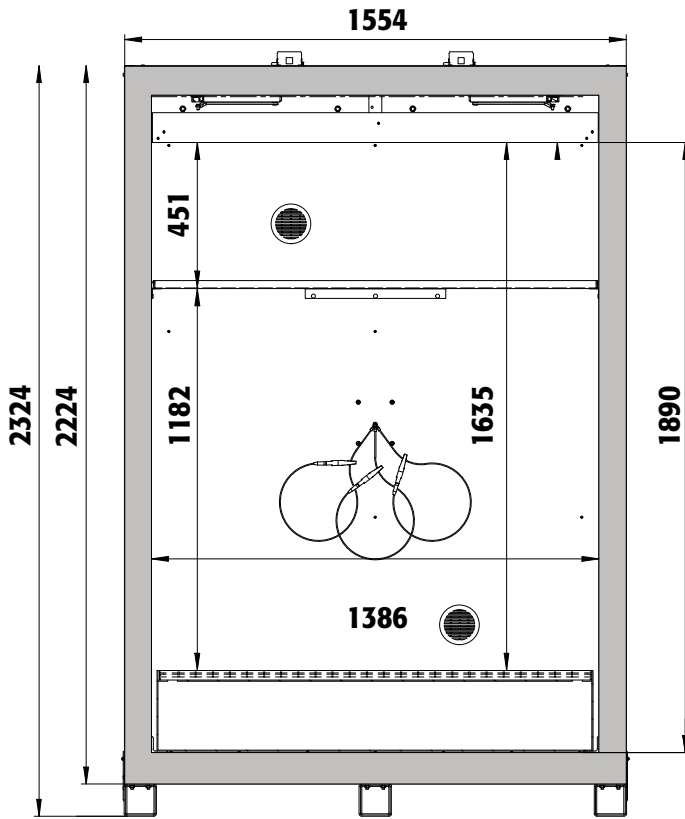
Vooranzicht
